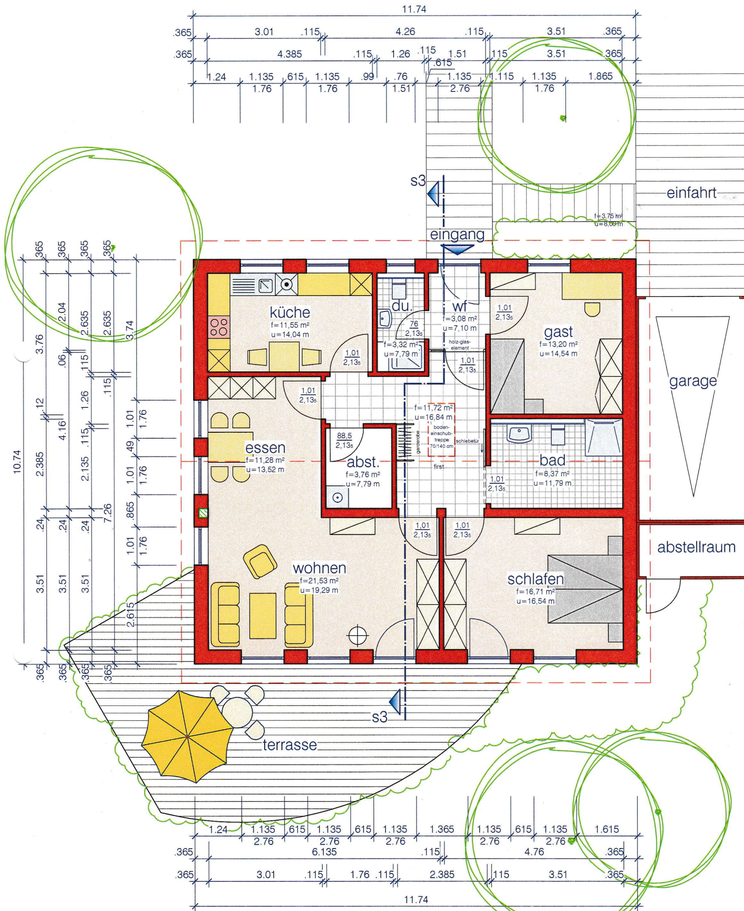
grundriss typ C
