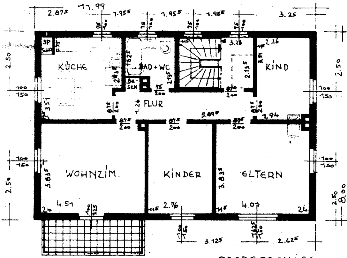
OBERGESCHOSS
